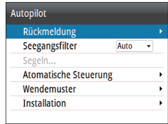
AC12N/AC42N – Einstellungen des Autopilot-Computers
