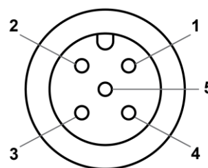
Micro-C M12 5-poliger Stecker Stecker, Kabelansicht
